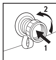
b) Poussez le bouchon de vidange et faites-le tourner dans le sens contraire des aiguilles d'une montre d'environ un quart de tour (90°) pour verrouiller
